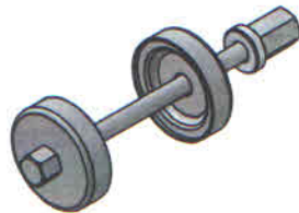
Ferramenta para colocar as buchas bipartida em aço da suspensão traseira Santana Versailles e Royale
