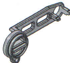
Ferramenta para sincronizar as polias das árvores de comando de válvulas dos motores VW EA211 1.0 12V MPI (3cil.) e 1.6 16V MSI.
