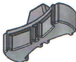
Ferramenta para sincronizar as polias das árvores de comando de válvulas do motor AT 1.0 16V (aspirado ou turbo) do Gol, Parati e Polo Classic
