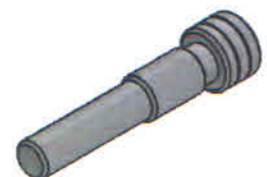
Pino para sincronizar a árvore de manivelas dos motores VW EA211 1.0 12V MPI (3cil.), 1.0 12V TSI (3cil.), 1.4 16V TSI/TFPI e Audi 1.6 16V MSI
